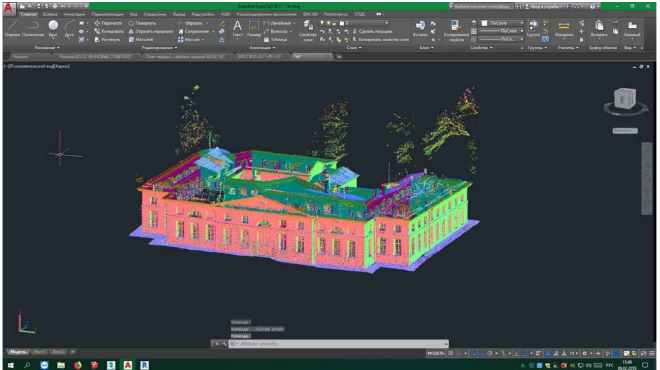
1. Облако точек – результат лазерного сканирования
