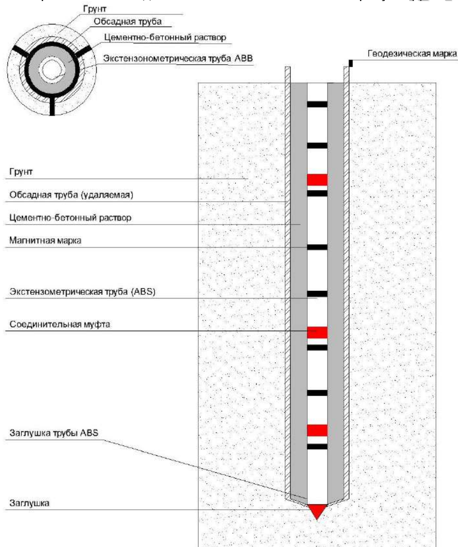
Рисунок Д.2 – Схема экстензометрической наблюдательной скважины
