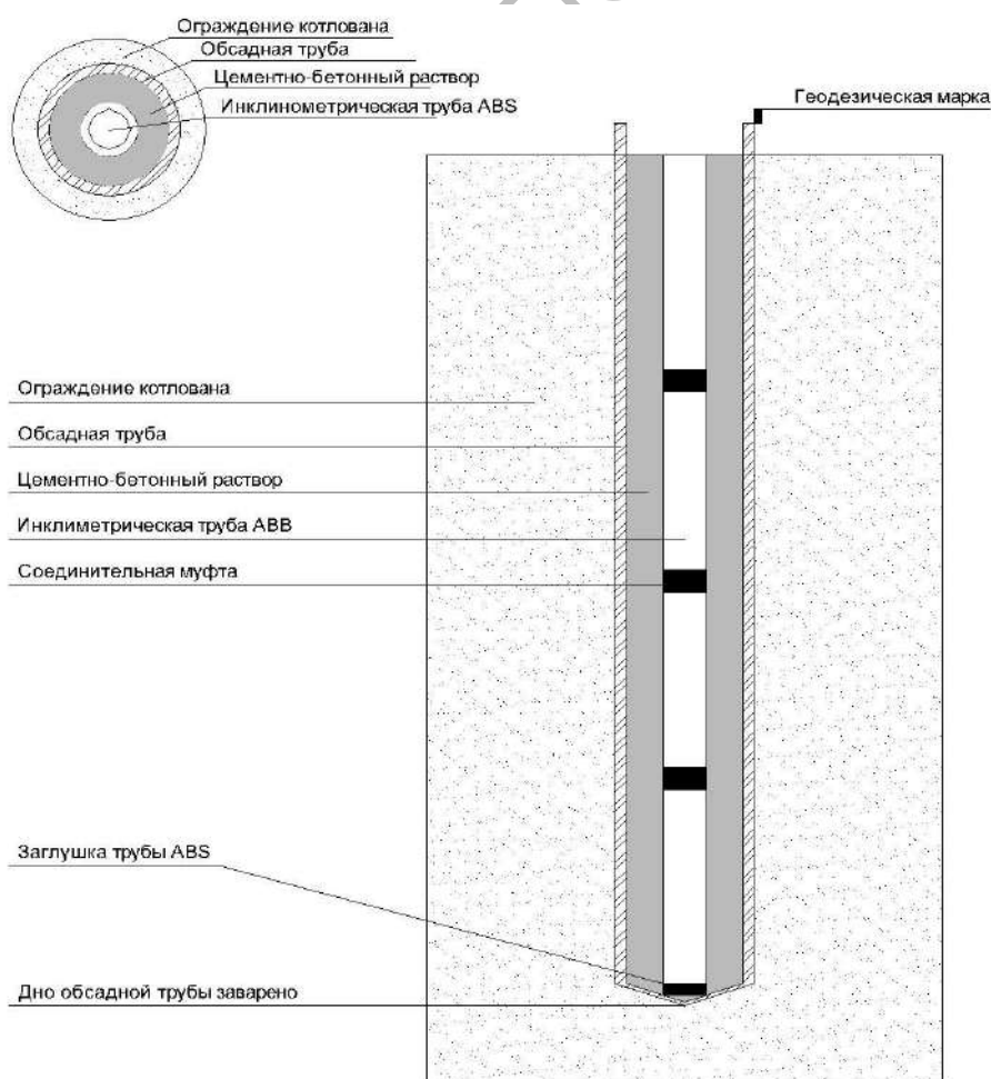
Рисунок Д.1 – Схема инклинометрической наблюдательной скважины
